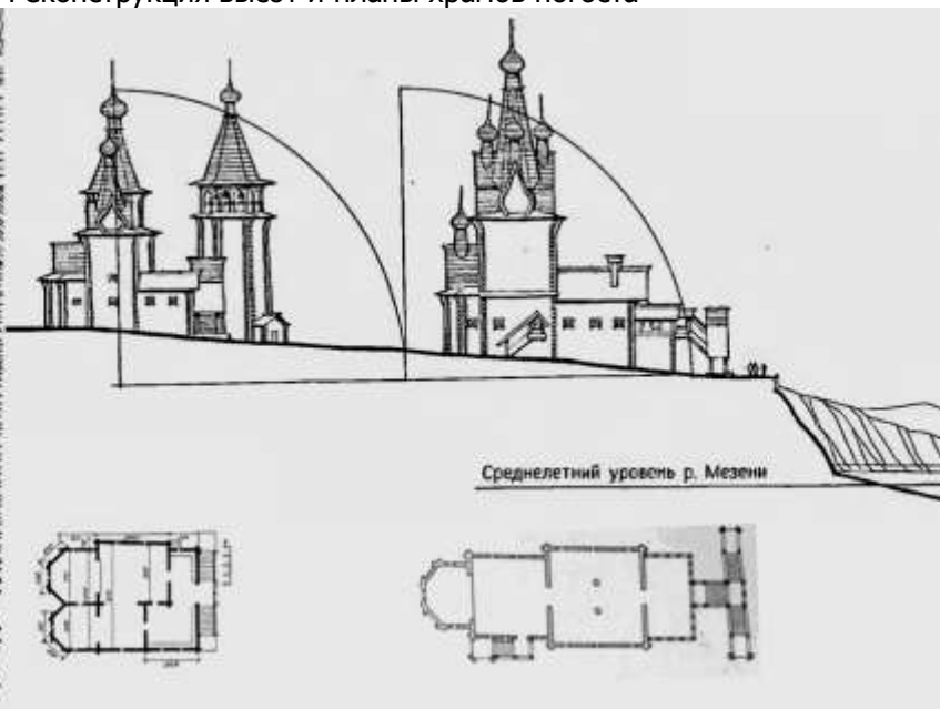
Реконструкция высот и планы храмов погоста
