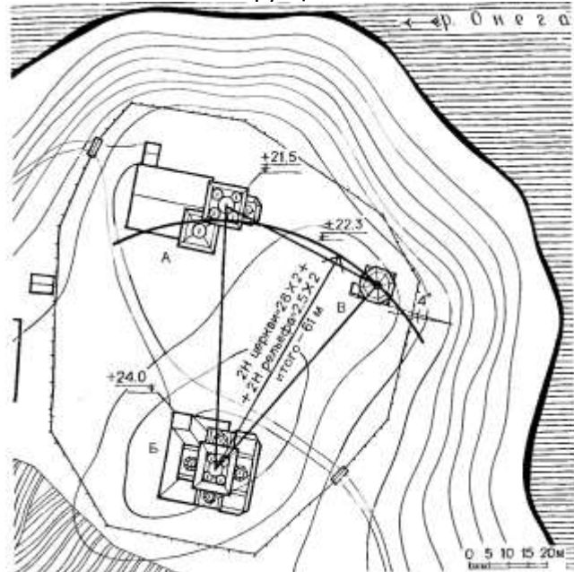
План погоста. Реконструкция Ю.С.Ушакова
