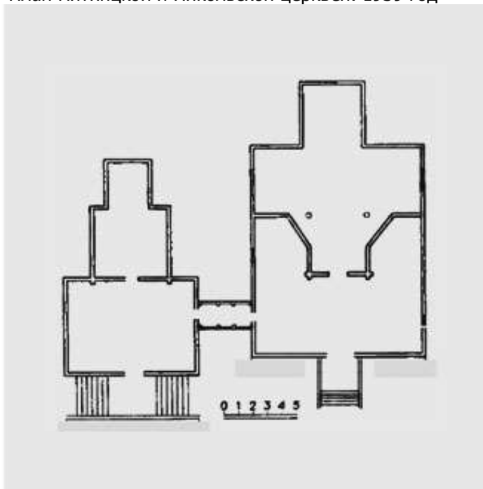
План Пятницкой и Никольской церквей. 1939 год
